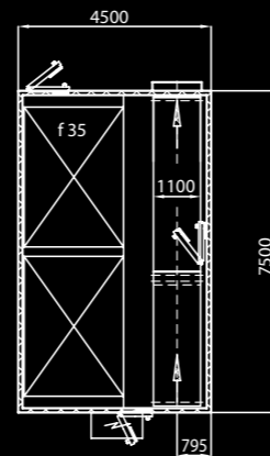
Компоновка f 35
