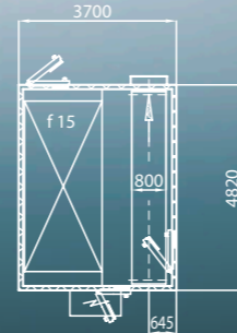
Компоновка f 15
